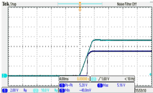
图 5: CH1 = 输出电压, CH3 = 额定输入电压 典型启动波型(满载)
