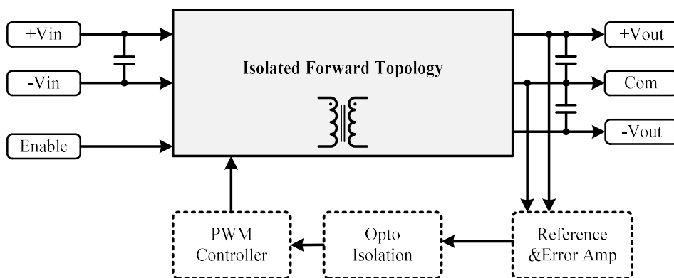
ESB 正负双路电路图
