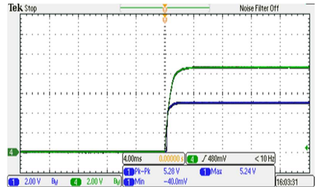
图 6: CH1 = 输出电压, CH3 = 远程遥控电压 典型启动波型(已设定输入电压)
