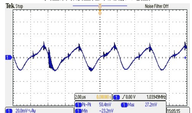
图 8: 出输出电压纹波与噪声(满载). (典型输入, 于输出端加 1uF MLCC 陶瓷电容)
