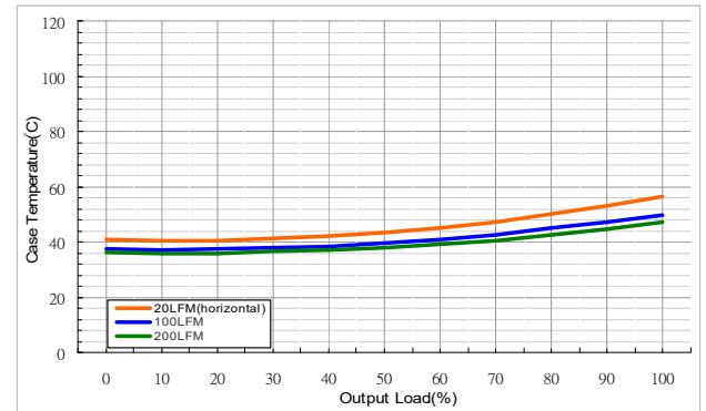
图 4: 工作壳温 VS 输出负载(满载)
